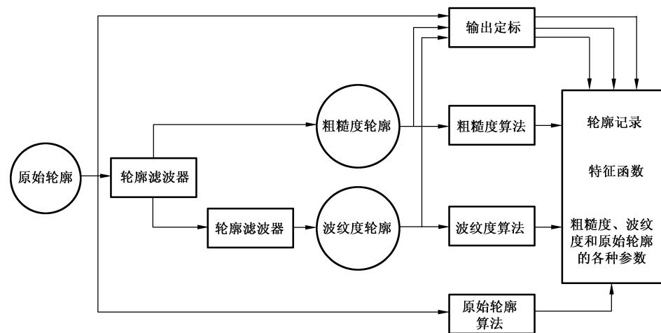
图 B.1 表面评定的流程图
